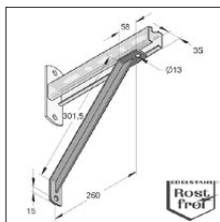
Zastrzał – 45° -T-Profil
